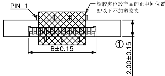
有凹槽舌片图示 SCALE 1:2
